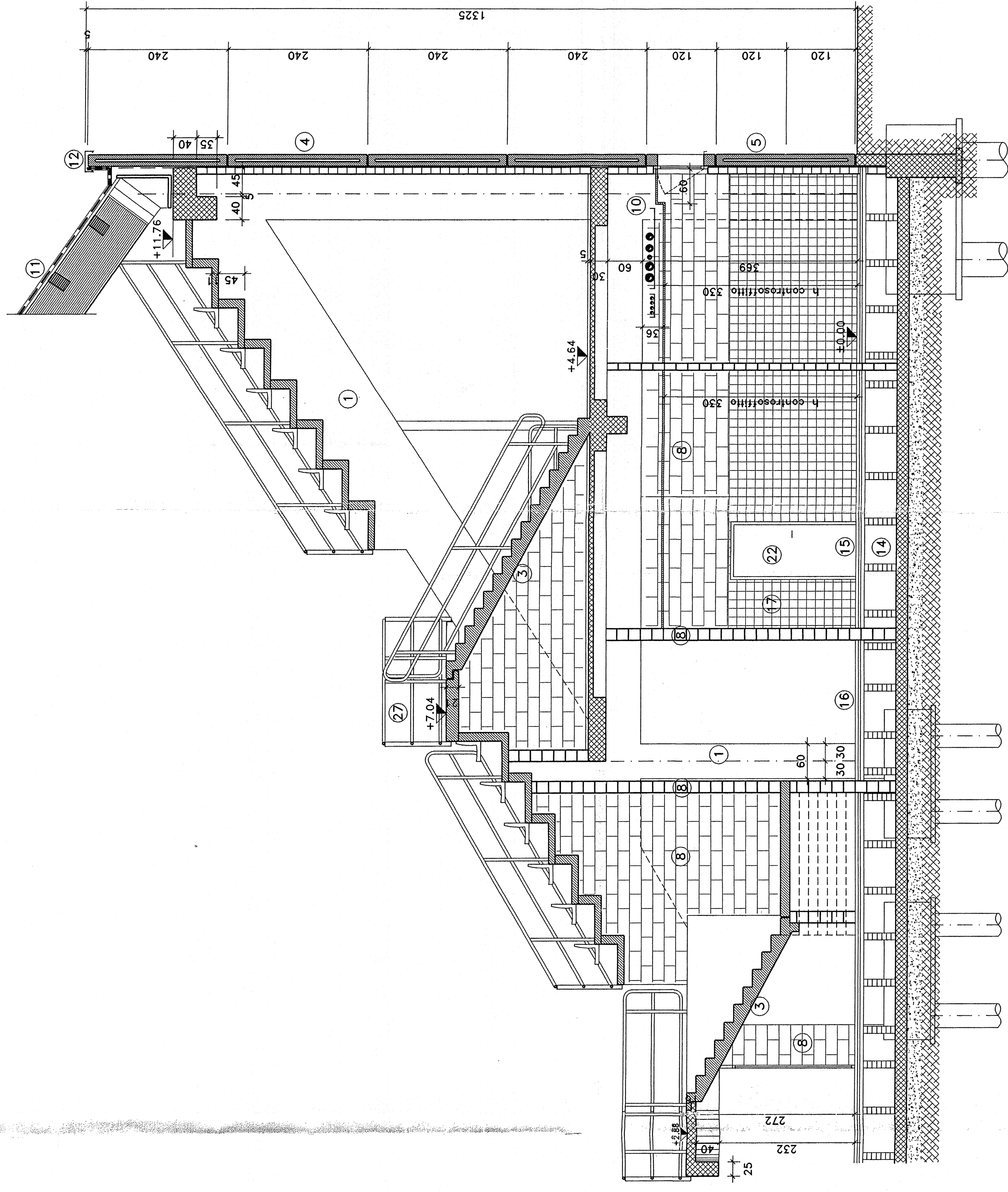
SEZIONE assi 19/20
