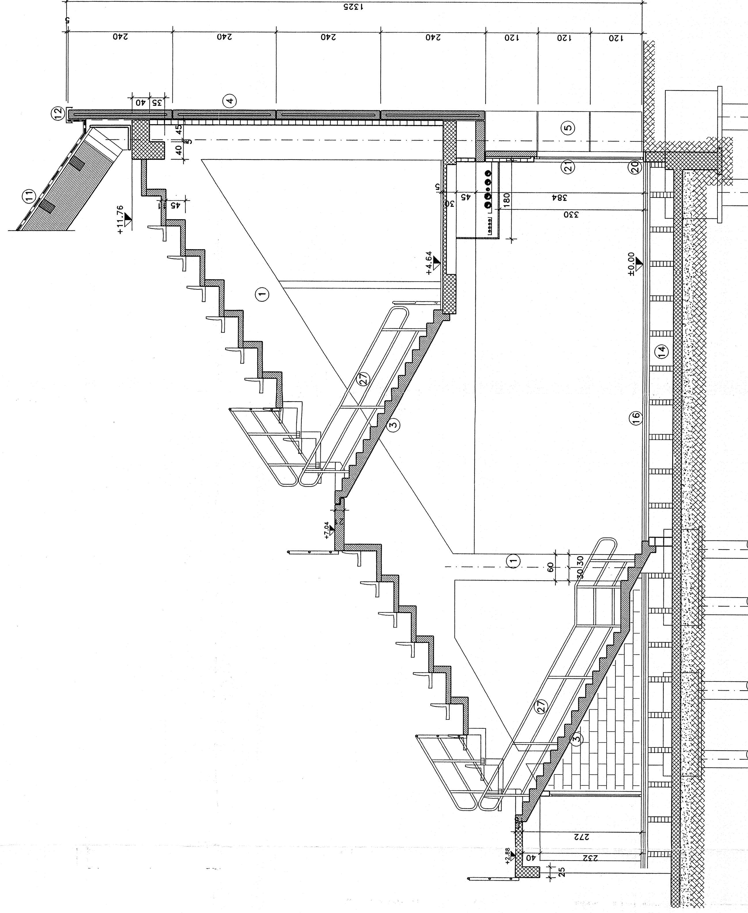
SEZIONE assi 26/27
